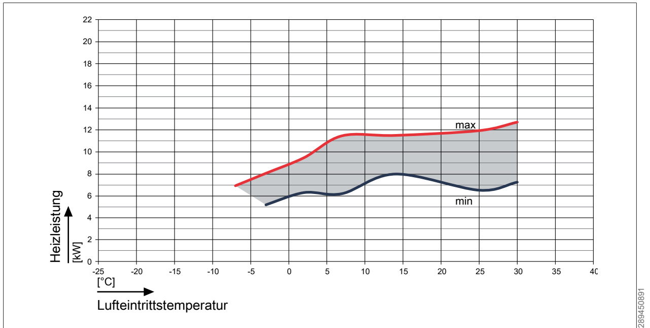
Abb. 58: Heizleistung FHA-14/17-400V bei einem Vorlauf von 60 ( \pm 2 ) °C
