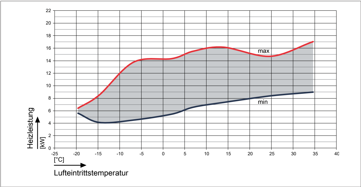
Abb. 48: Heizleistung FHA-14/17-230V bei einem Vorlauf von 35 °C
