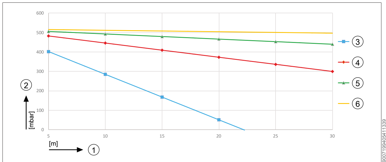
Abb. 4: FHA-08/10 Verfügbare Förderhöhe
