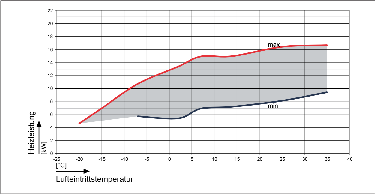
Abb. 49: Heizleistung FHA-14/17-230V bei einem Vorlauf von 45 °C
