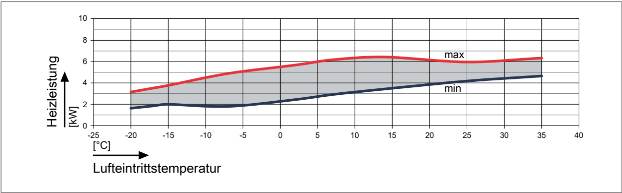
Abb. 13: Heizleistung FHA-05/06 bei einem Vorlauf von 35 °C
