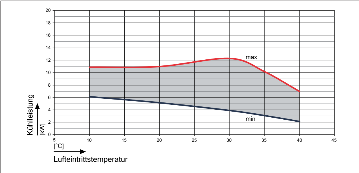
Abb. 39: K hlleistung FHA-11/14-230V bei einem Vorlauf von 7  C
