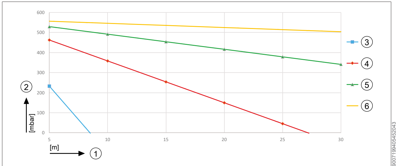
Abb. 6: FHA-14/17 Verfügbare Förderhöhe
