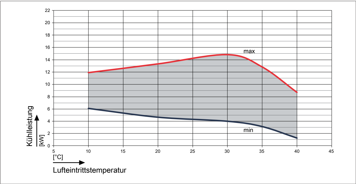
Abb. 60: Kühlleistung FHA-14/17-400V bei einem Vorlauf von 7 °C
