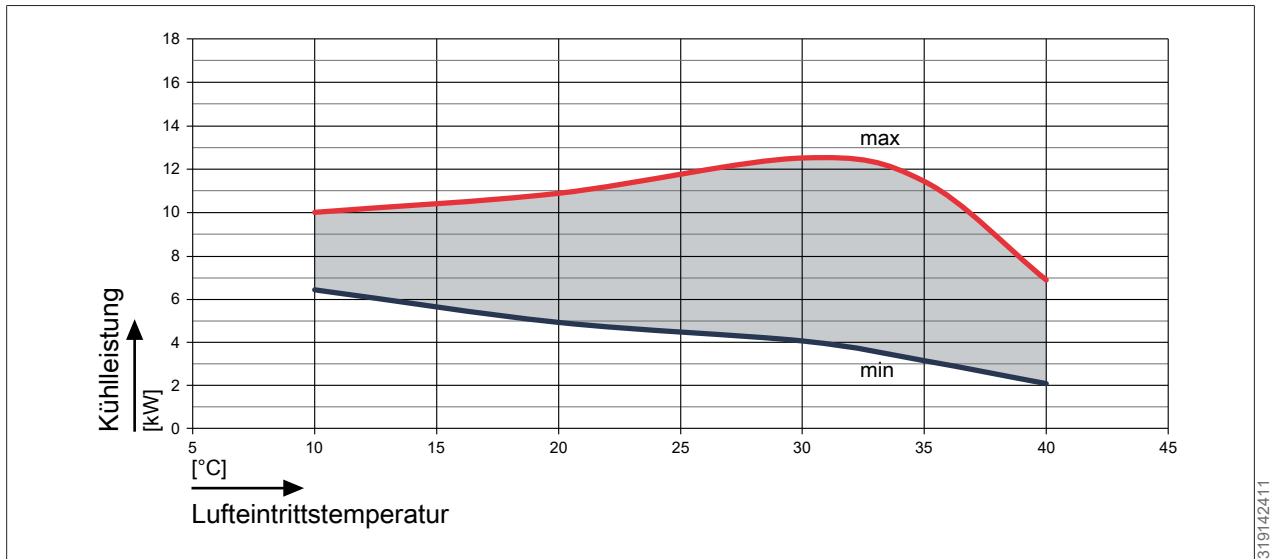
Abb. 46: Kühlleistung FHA-11/14-400V bei einem Vorlauf von 7 °C
