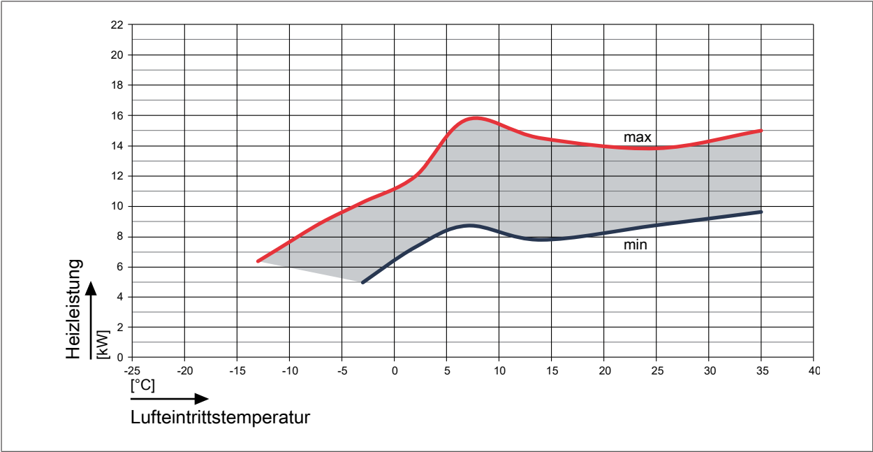
Abb. 57: Heizleistung FHA-14/17-400V bei einem Vorlauf von 55 °C
