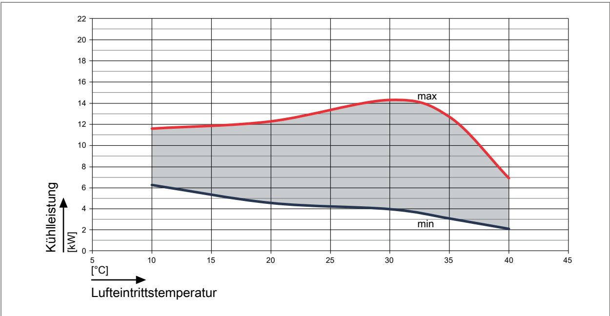
Abb. 53: Kühlleistung FHA-14/17-230V bei einem Vorlauf von 7 °C
