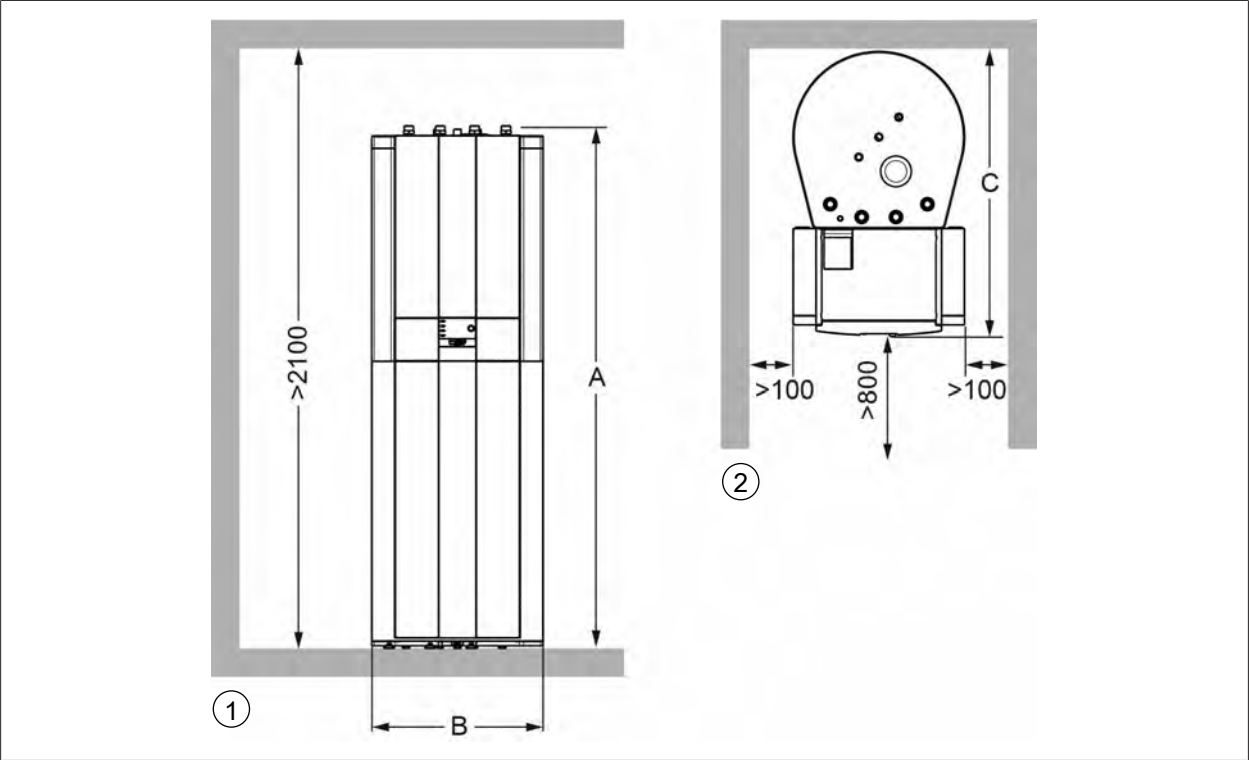
1 Vorderansicht FHA-Center 300 2 Draufsicht FHA-Center 300
