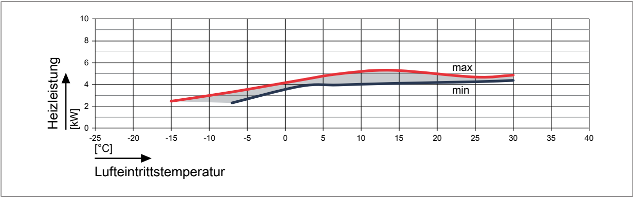
Abb. 16: Heizleistung FHA-05/06 bei einem Vorlauf von 60 (± 2) °C
