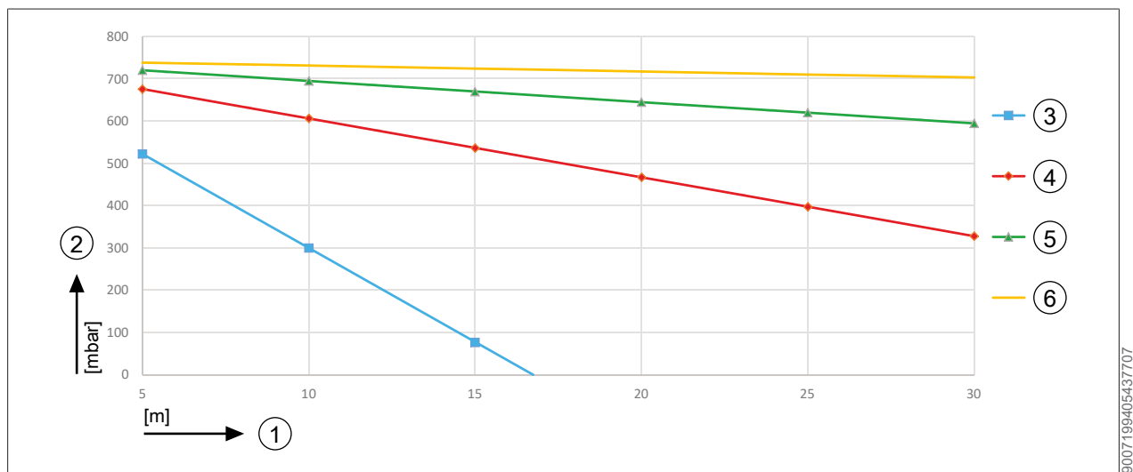
Abb. 5: FHA-11/14 Verfügbare Förderhöhe
