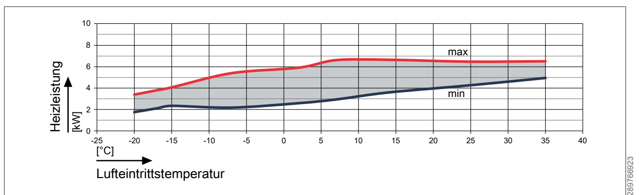
Abb. 12: Heizleistung FHA-05/06 bei einem Vorlauf von 25 °C
