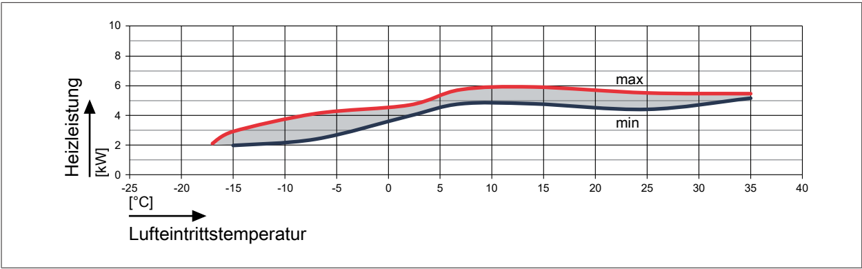
Abb. 15: Heizleistung FHA-05/06 bei einem Vorlauf von 55 °C
