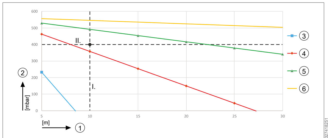
Abb. 1: FHA-14/17 Verfügbare Förderhöhe
