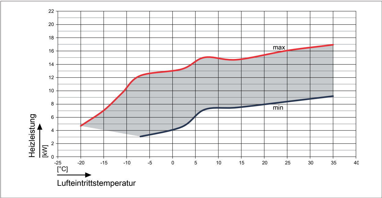
Abb. 56: Heizleistung FHA-14/17-400V bei einem Vorlauf von 45 °C
