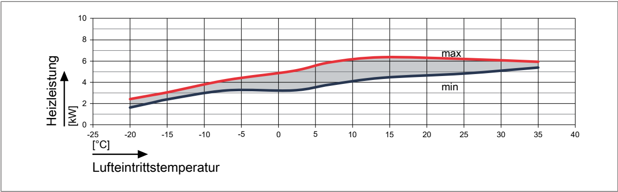
Abb. 14: Heizleistung FHA-05/06 bei einem Vorlauf von 45 °C
