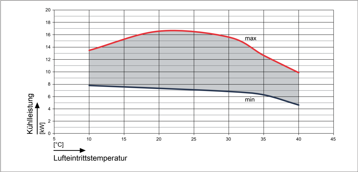
Abb. 38: K hlleistung FHA-11/14-230V bei einem Vorlauf von 18  C
