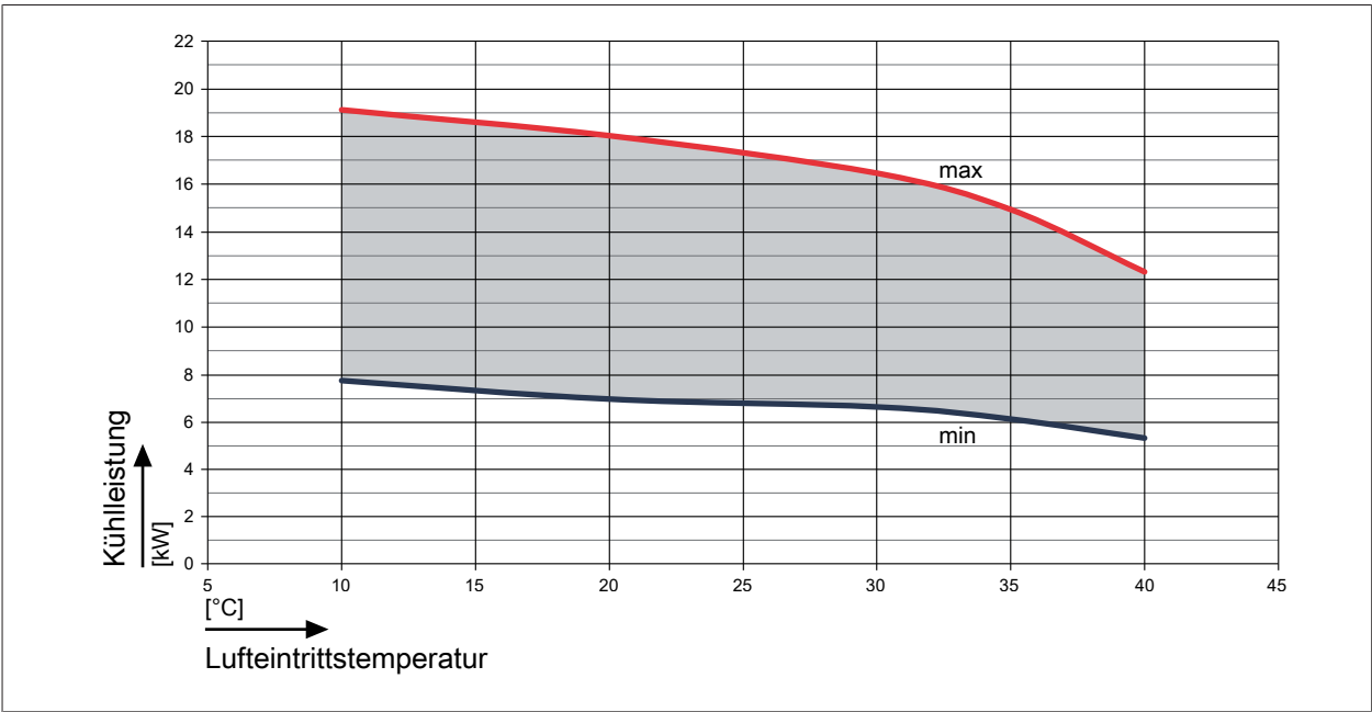
Abb. 52: Kühlleistung FHA-14/17-230V bei einem Vorlauf von 18 °C
